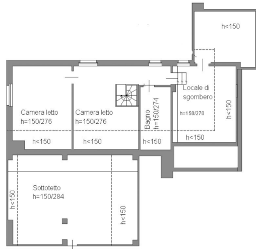
PIANO PRIMO (SOTTOTETTO)
